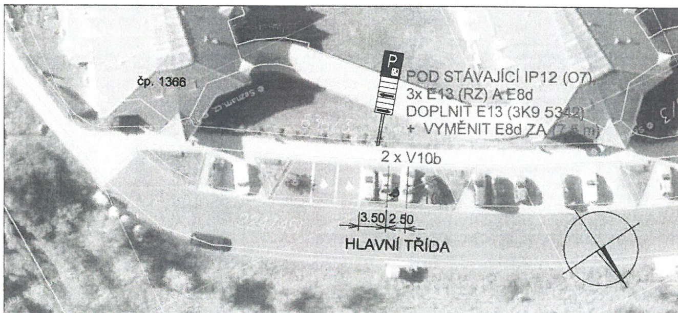
Obr. č. 7 – Situace 1 : 500:
